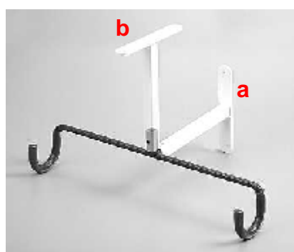
konzola v polohe upevnenia (a) na stenu (b) na strop
